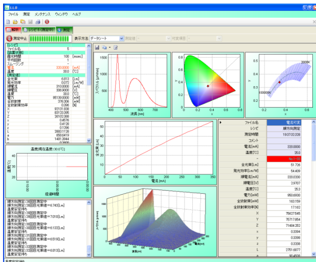
電流可変データ
