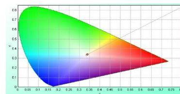
色度図
