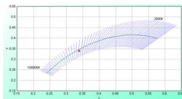
色温度図
