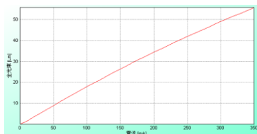
全光束-電流グラフ
