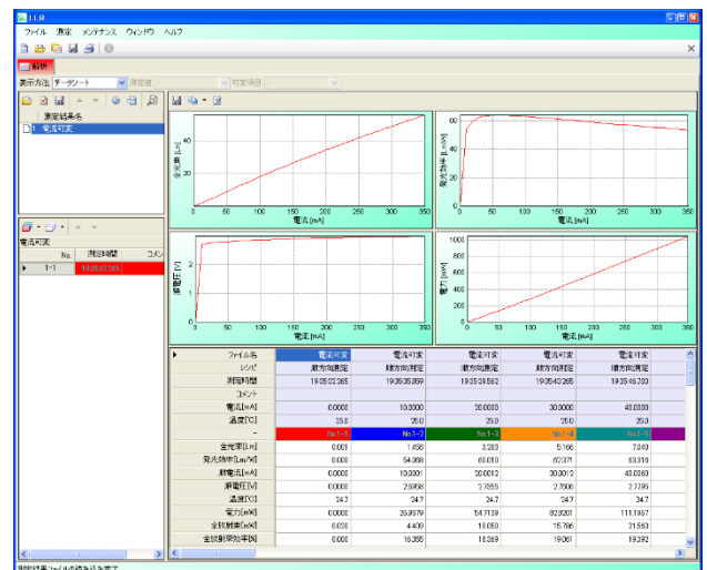
温度可変データ
